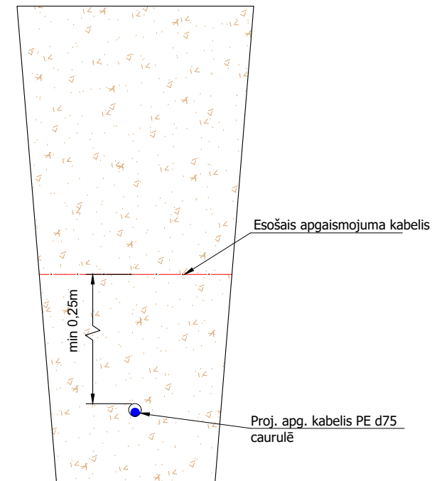
Proj. pēcuskaites kabeļa šķērsojums ar apgaismojuma kabeli
