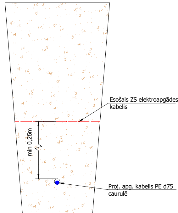
Proj. pēcuskaites kabeļa šķērsojums ar ZS elektroapgādes kabeli
