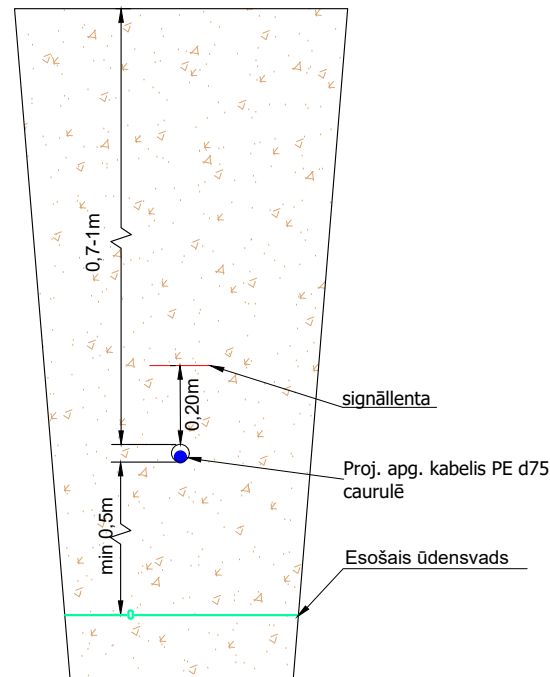
Proj. pēcuskaites kabeļa šķērsojums ar esošo ūdensvadu
